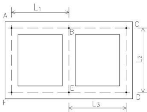
走道防烟分区长边长度： L_{\max} = L_{AD} = L_1 + L_2 + L_3
