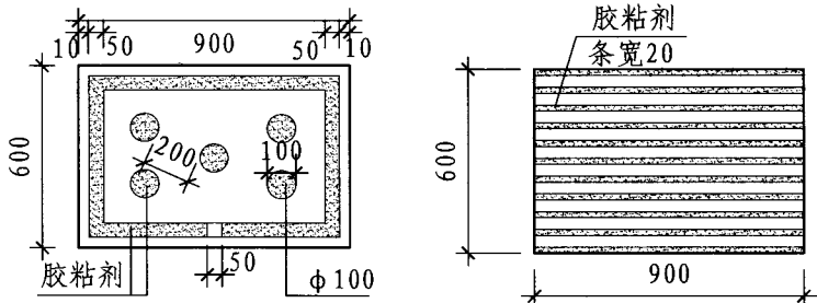
图B-2 点框粘法示意图 图B-3 条粘法示意图
