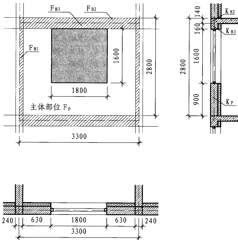
外墙主体部位与周边热桥部位示意
