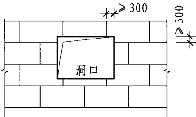
图B-1 门窗洞口保温板排列
