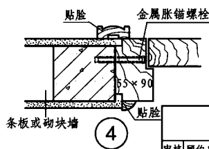
木框装饰门立口详图
