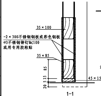
门扇包钢护板大样 (用于医院)
