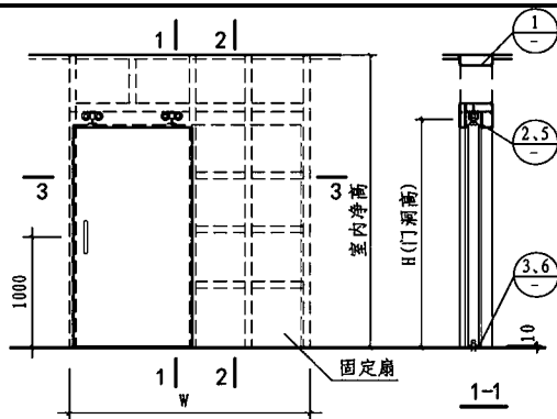
单扇明装推拉门立面图
