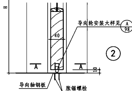
单扇暗装推拉门安装图
