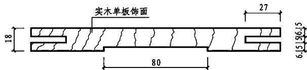
双线带上亮平开门套立挺、冒头
