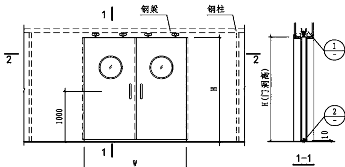
双扇暗装推拉门立面图
