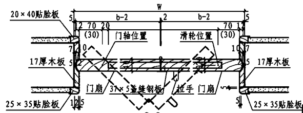
双扇折叠门平面放大图
