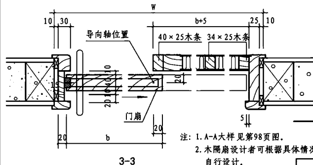
单扇明装推拉门平面放大图
