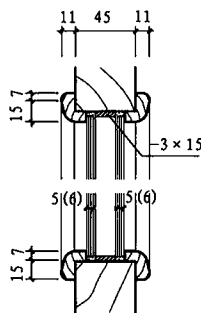
3-3 双玻铁艺门
