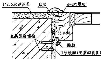
① 用于混凝土墙或砌块墙
