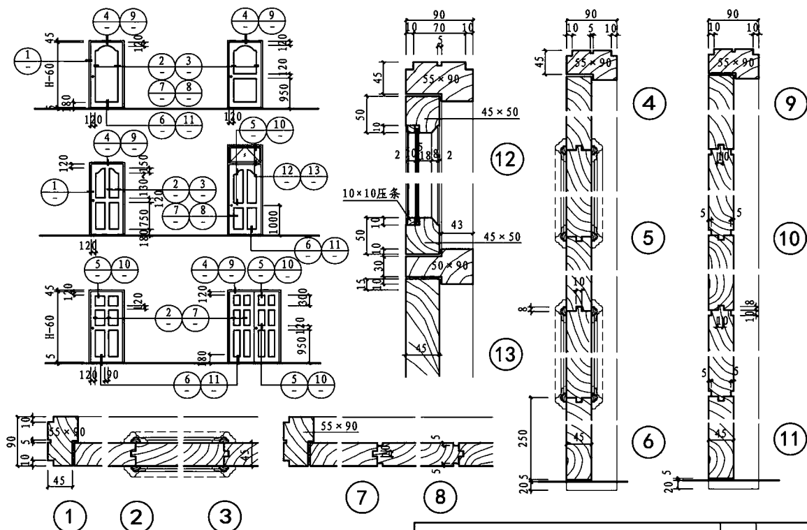
木框平开装饰门节点详图
