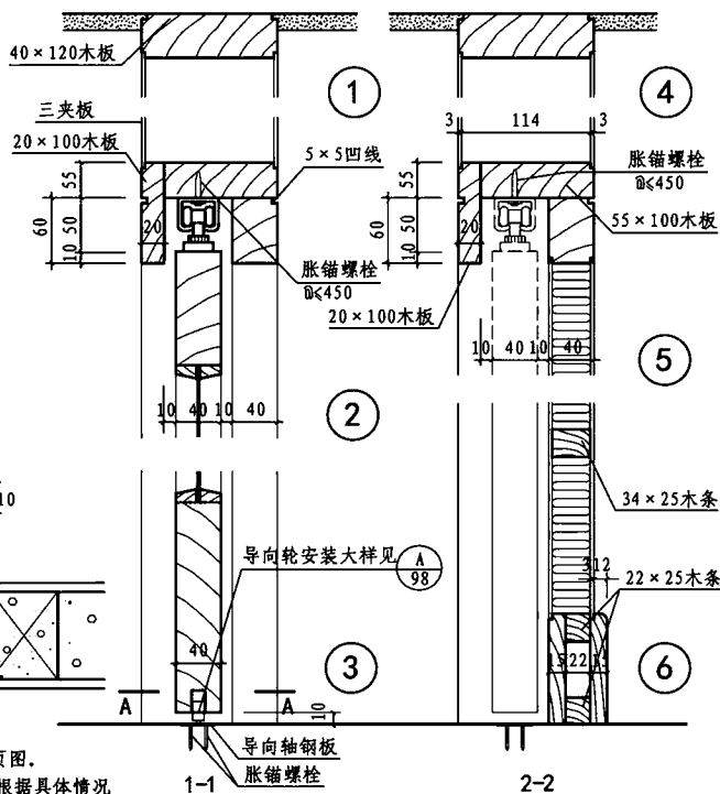
100厚轻质墙上推拉门安装图
