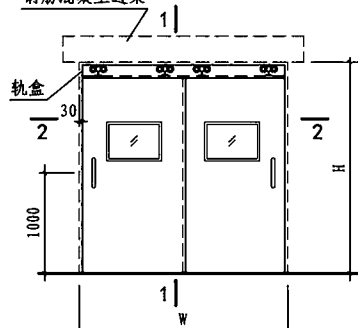
双扇明装推拉门立面图
