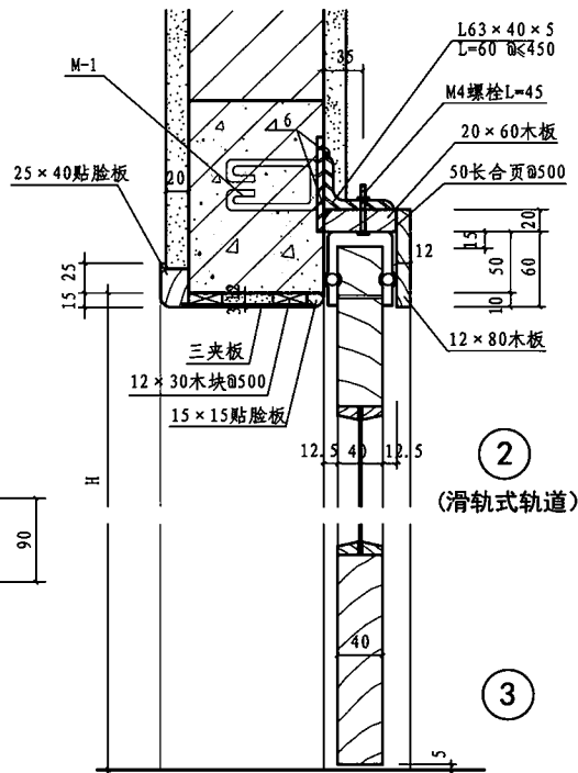
滑轨式和上挂式明装推拉门连接件及大样
