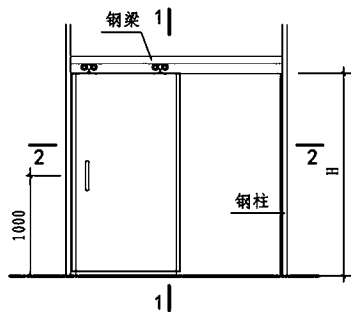
单扇暗装推拉门立面图
