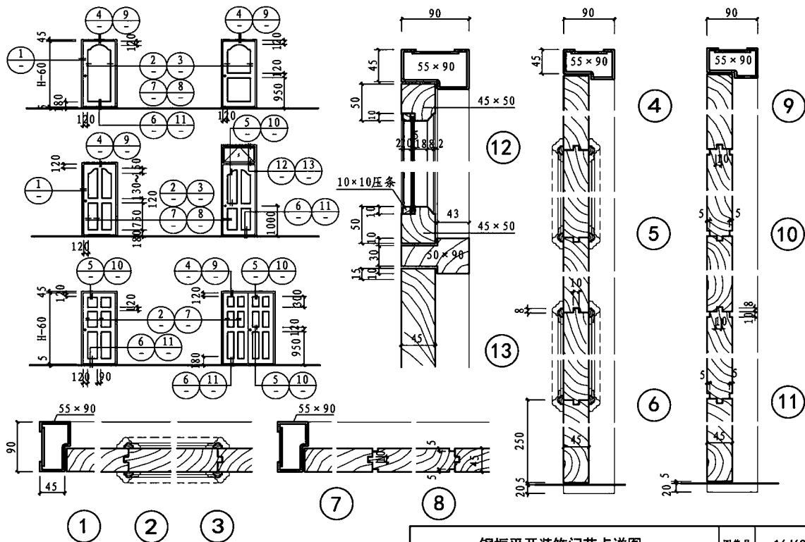
钢框平开装饰门节点详图
