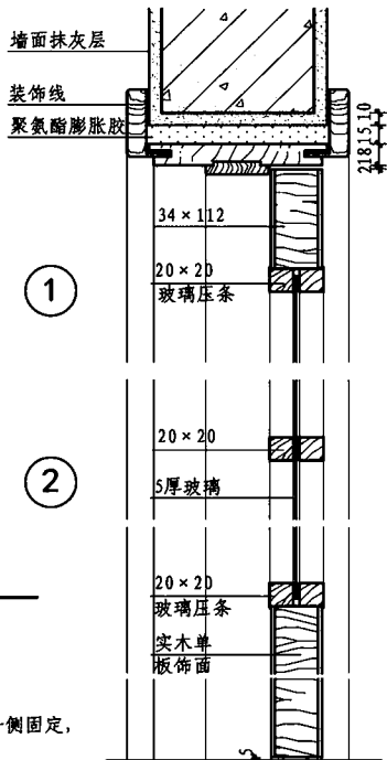
板框镶玻璃门节点详图
