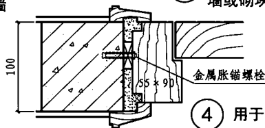
木框平开门安装图
