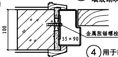
钢框平开门安装图
