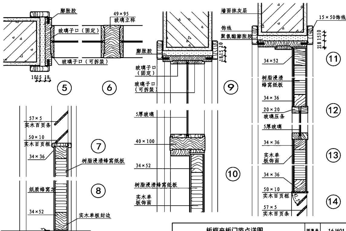
板框夹板门节点详图
