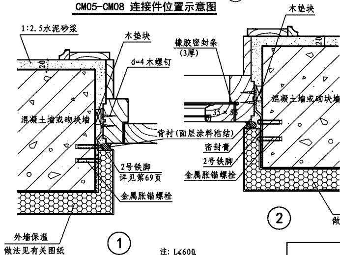
CM05-CM08 连接件位置示意图
