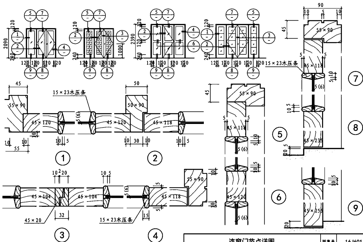
连窗节点详图
