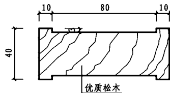
平开门套上亮横档
