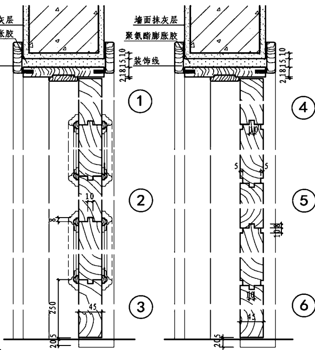
板框平开装饰门节点详图
