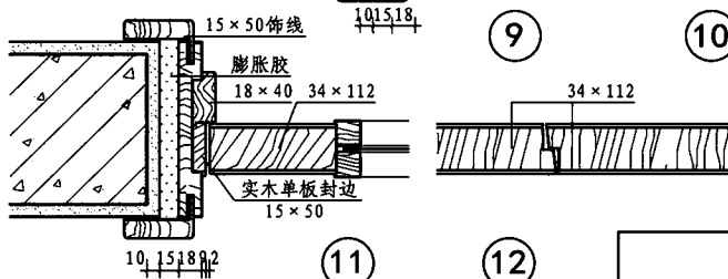
板框镶玻门节点详图
