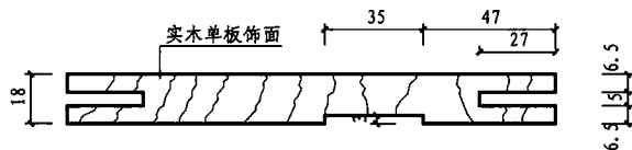
双线平开门套立挺、冒头
