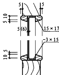
2-2 单玻铁艺门
