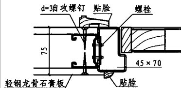
③ 用于轻钢龙骨石膏板
