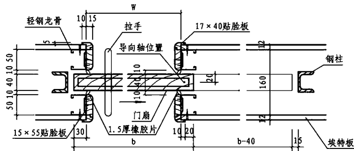
单扇暗装推拉门平面放大图
