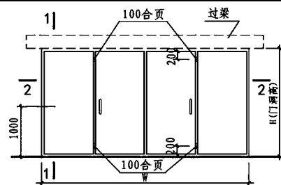
四扇折叠门立面图
