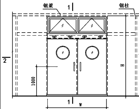
双扇暗装推拉门立面图
