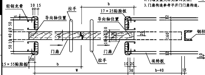
双扇暗装推拉门安装图
