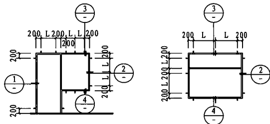
CM05-CM08 连接件位置示意图
