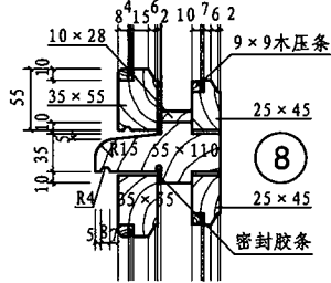
带纱扇平开外窗节点详图
