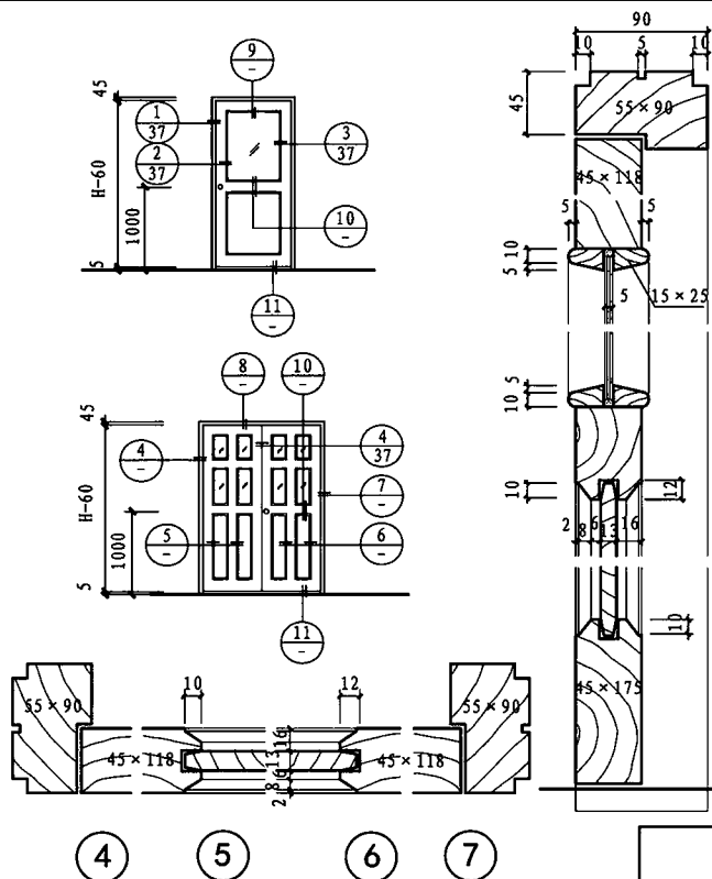
木框镶玻璃门节点详图
