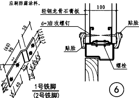
钢框装饰门立口详图
