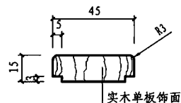
子口
