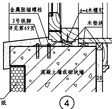
连窗门安装图
