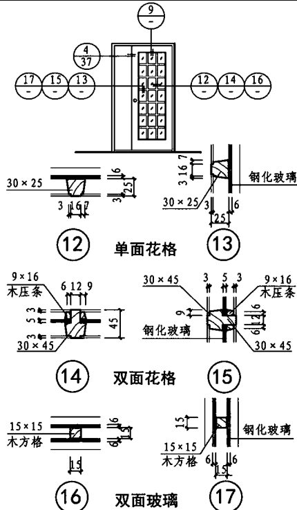
木框镶玻璃门节点详图
