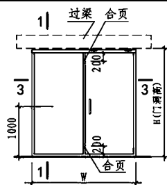
二扇折叠门立面图
