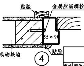
钢框装饰门立口详图
