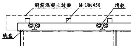
单扇明装推拉门上挂式滑轮安装示意图
