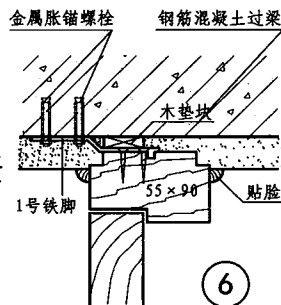
② 用于混凝土墙或砌块墙
