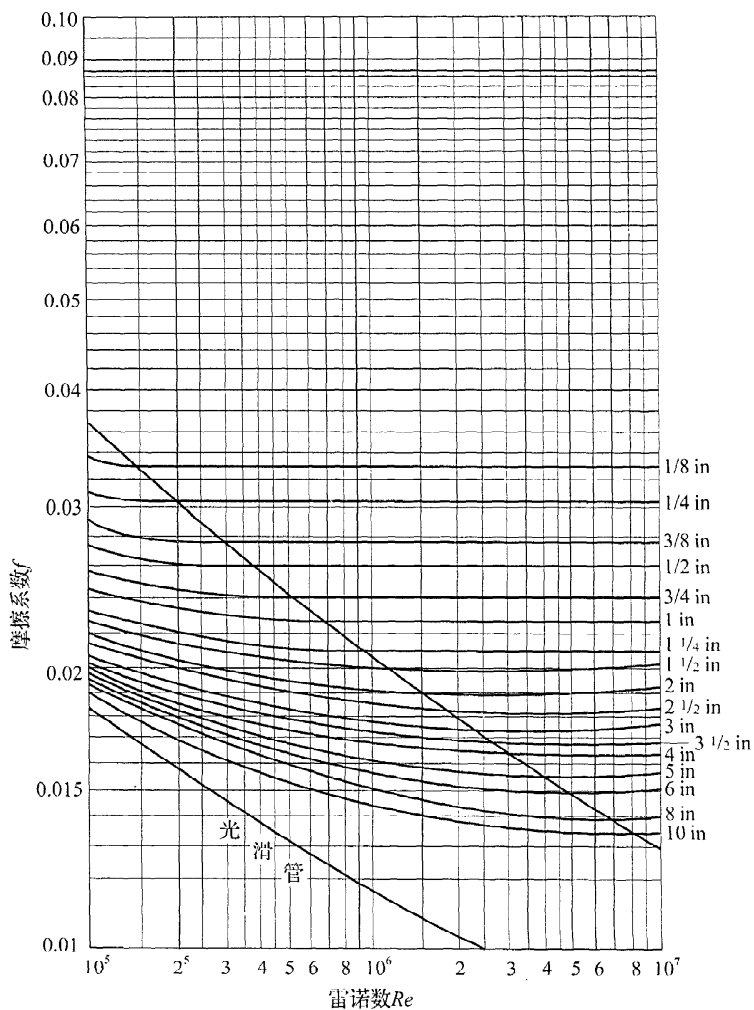
图 9 钢管莫迪图( Re \geq 10^5 )
