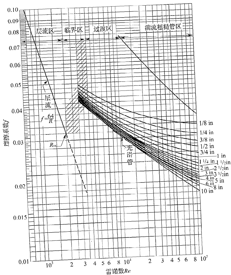
图 8 钢管莫迪图 ( Re \leq 10^5 )
