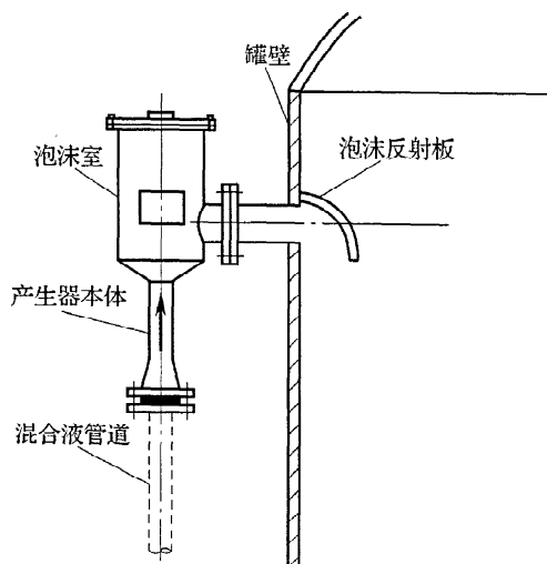
图 3 立式泡沫产生器安装示意
