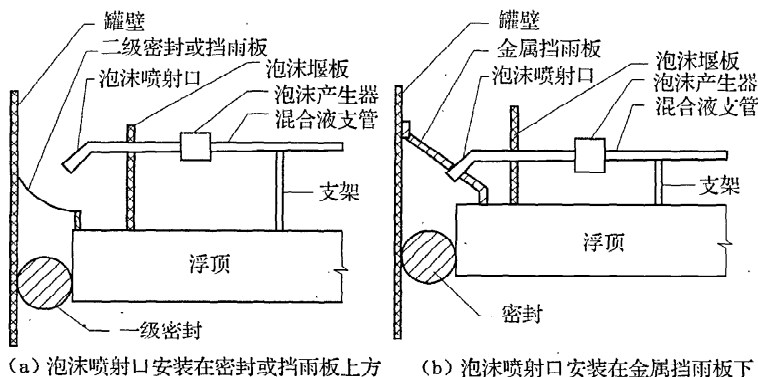
图6 泡沫喷射口在浮顶上的安装方式
