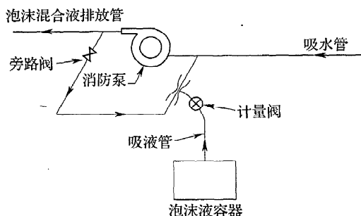
图 2 环泵式比例混流程示意
