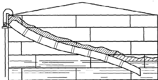
图5 泡沫溜槽
