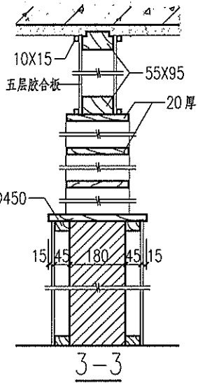
博古架木隔断 (一)
