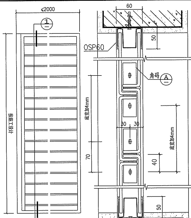
U玻横向安装立面
