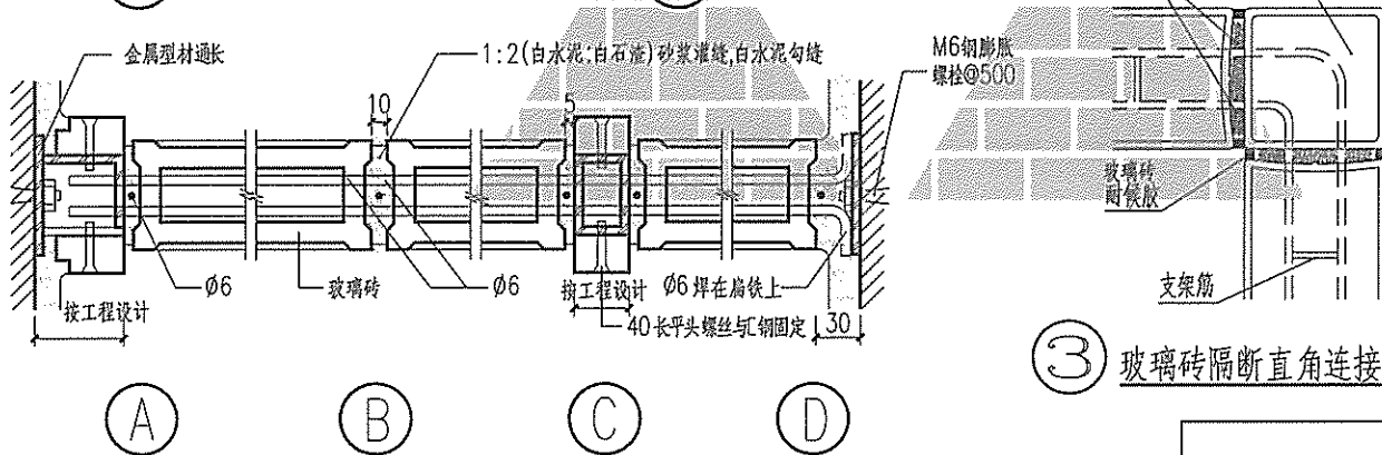
① 玻璃砖隔斷1型平面图
