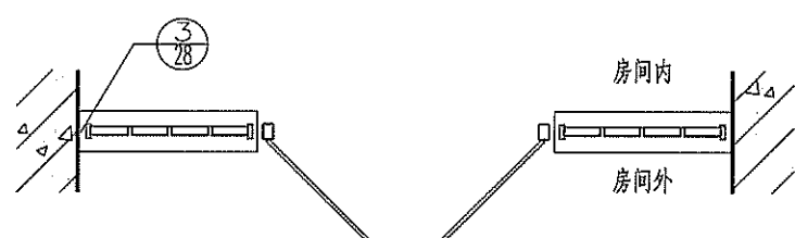
④ 单层全玻带门隔断平面图
