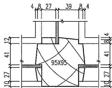
G 丁字连接
