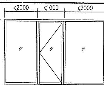
基本单元1与平开门组合立面示意图2
