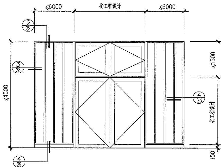
③ 单层全玻带门隔断立面图
