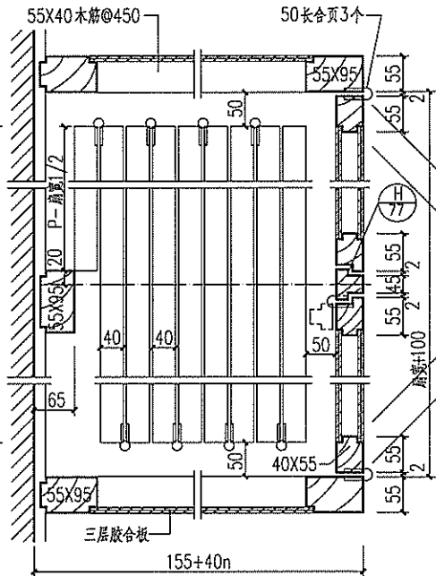
③ 平面图
