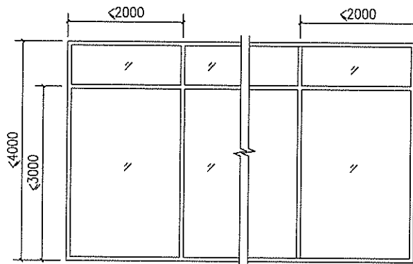
基本单元2组合立面示意图
