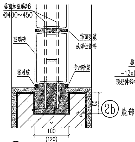
② 预留凹槽玻璃砖隔断做法
