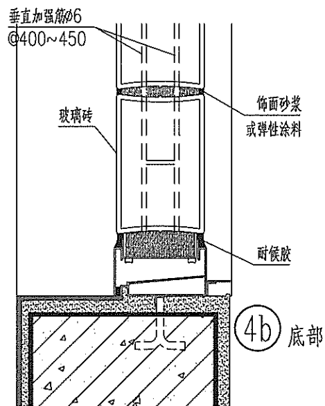
④ 有框玻璃砖隔断做法
