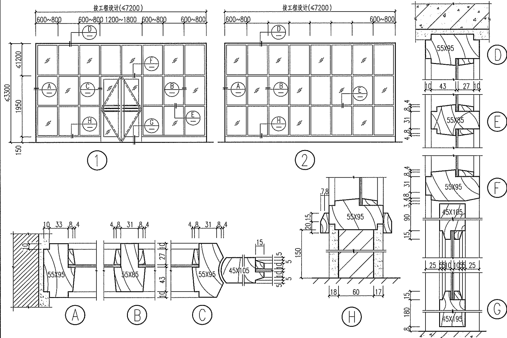
玻璃木隔断 (一)
