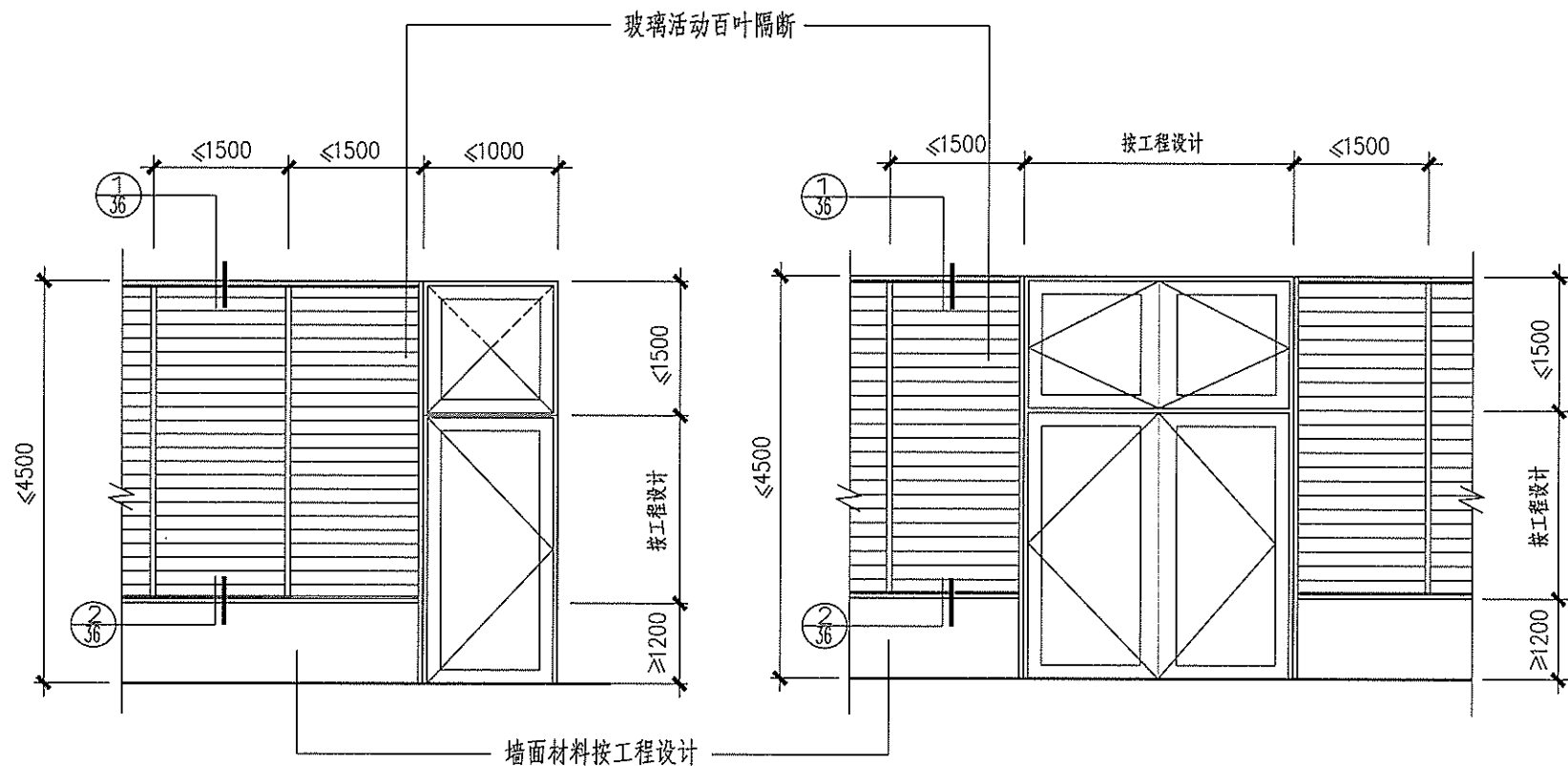
① 玻璃活动百叶隔断立面图
