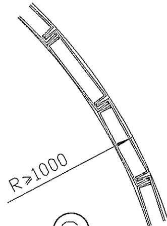
全玻弧形平面示意图
