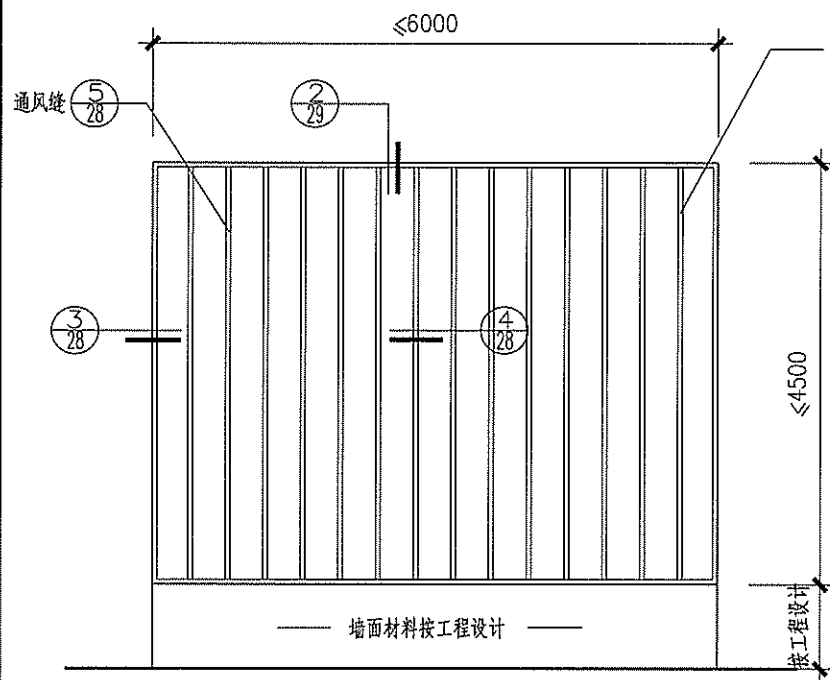
① 单层半玻隔断立面图
