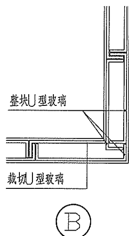
全玻转角裁切方式2
