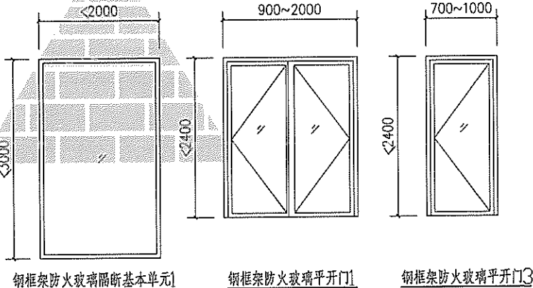
防火玻璃隔断说明(二)
