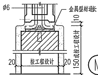
③ 玻璃砖隔断直角连接
