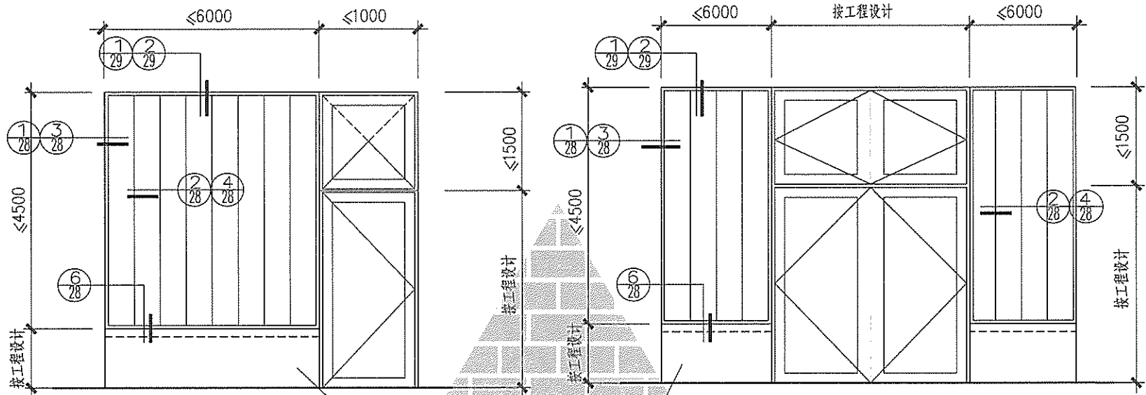
2 a 半玻带门隔断立面图
