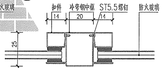
⑤ 隔断水平连接
