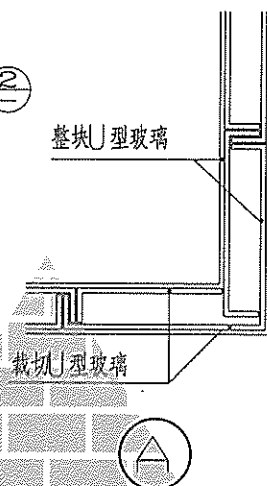
全玻转角裁切方式1
