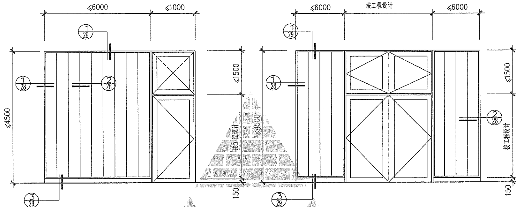
① 双层全玻带门隔断立面图
