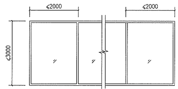
基本单元1 组合立面示意图
