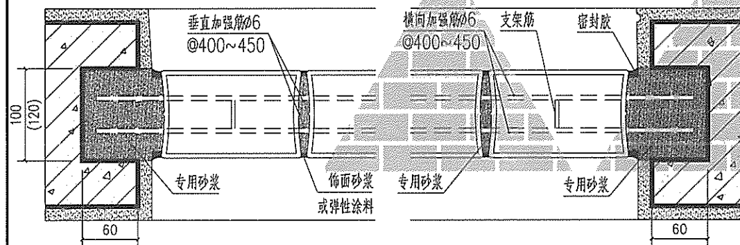
① 预留凹槽玻璃砖隔断做法平面
