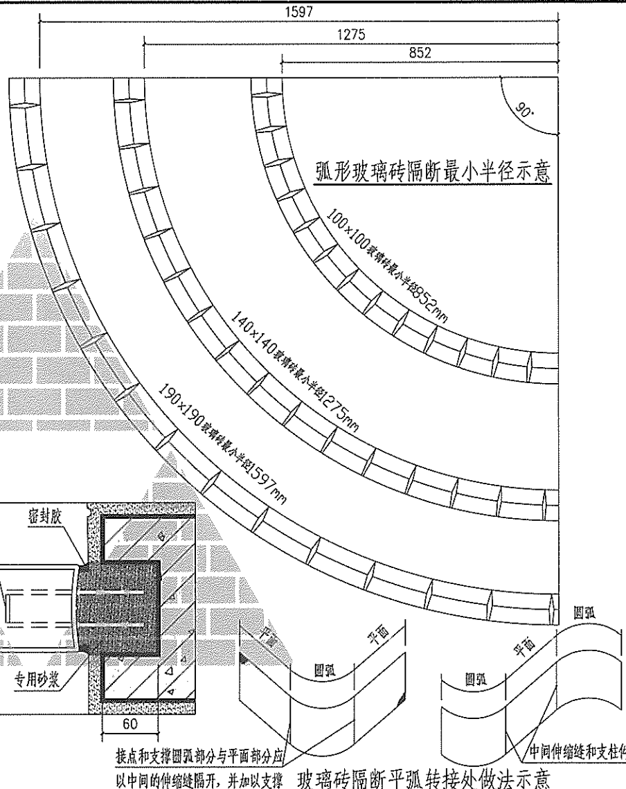
玻璃砖隔断 (一)
