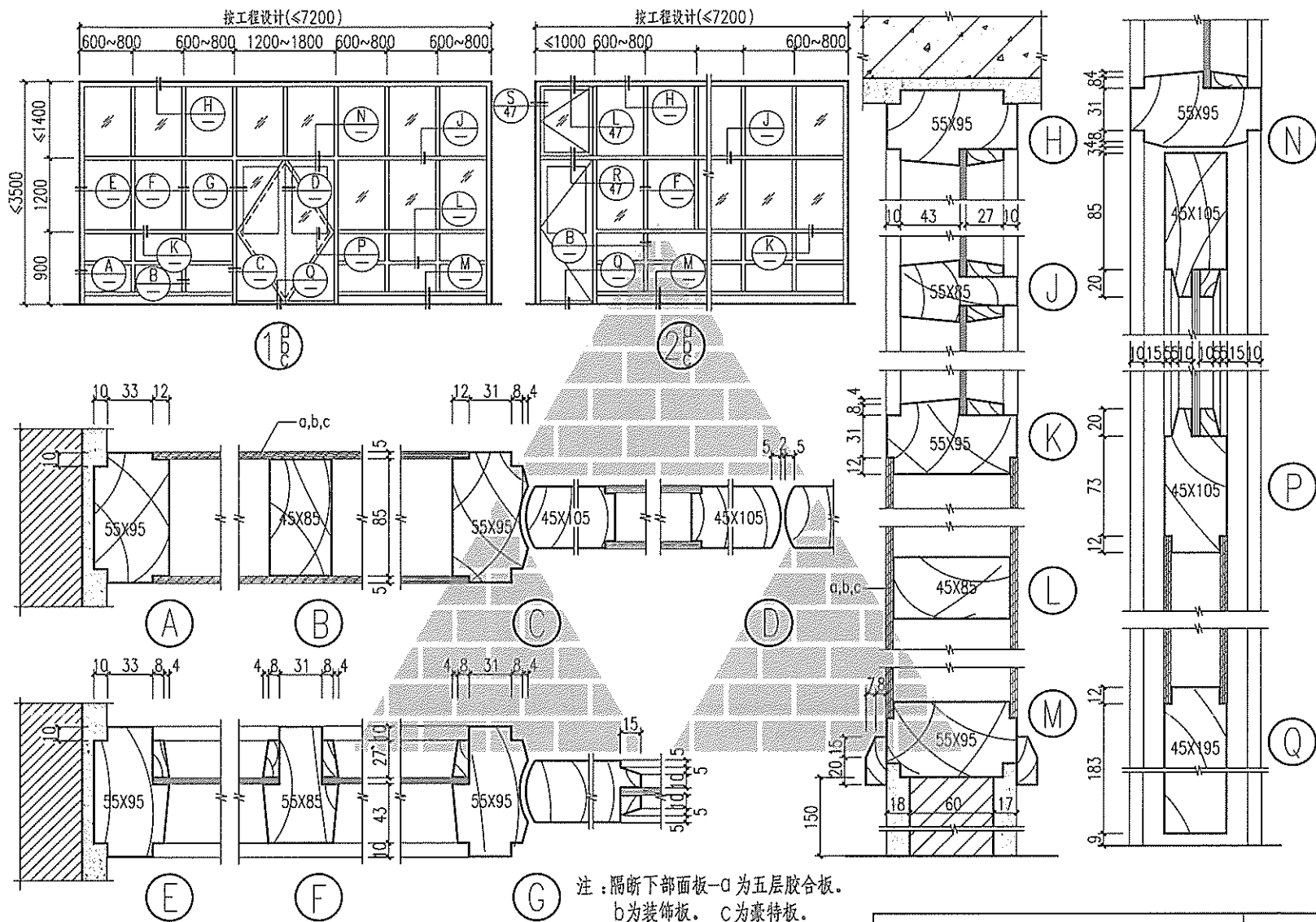
玻璃木隔断(二)
