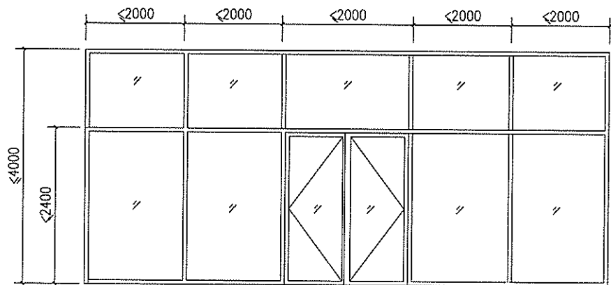
基本单元2与平开门组合立面示意图1
