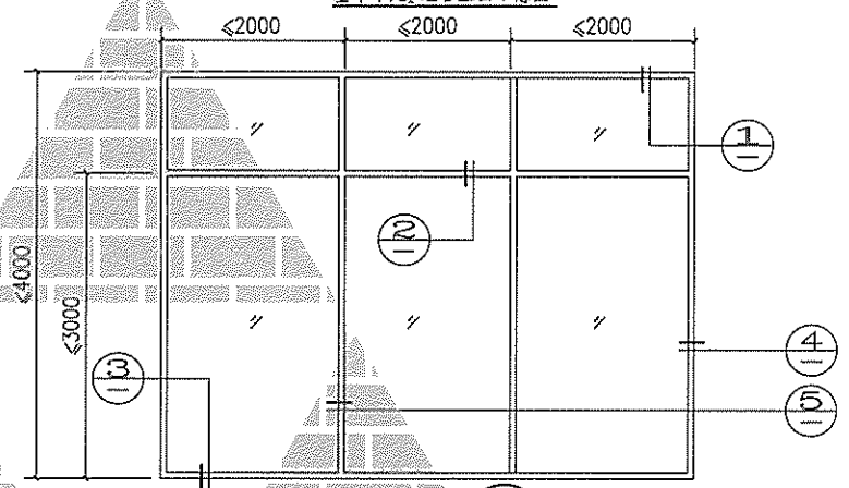
防火玻璃隔断立面图 A
