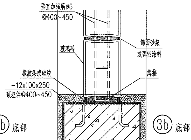
③ 预埋件玻璃砖隔断做法
