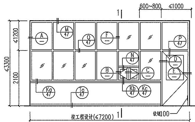
1-1 立面
