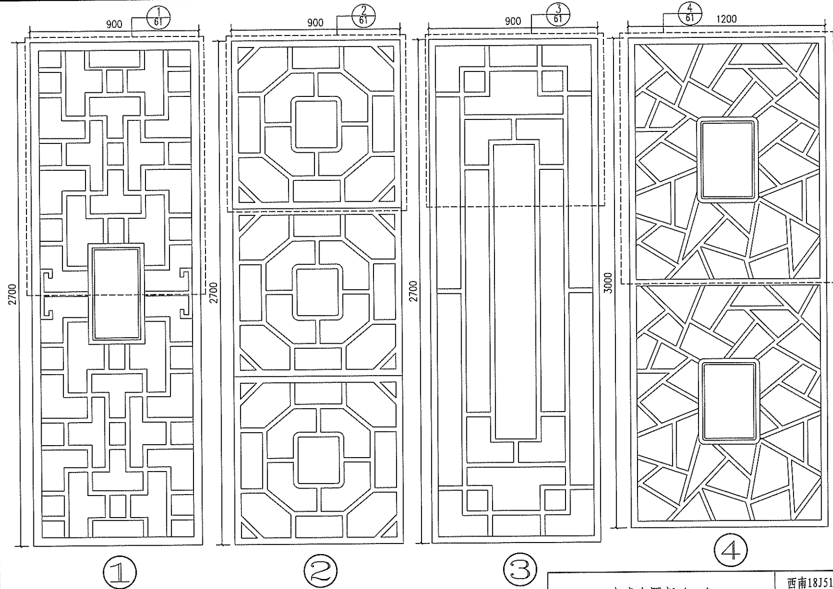
中式木隔断 (一)
