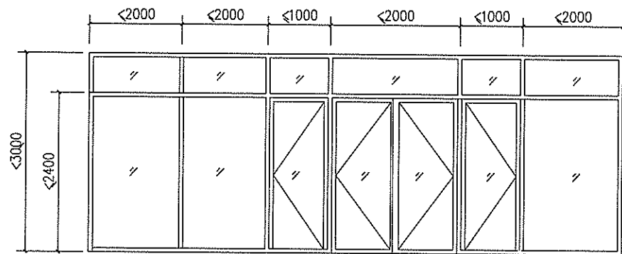
基本单元1与平开门组合立面示意图3
