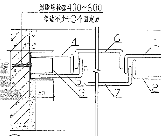
端头玻璃安装顺序 1、2为门窗端头
