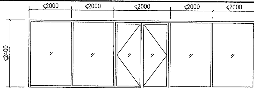
基本单元1与平开门组合立面示意图1
