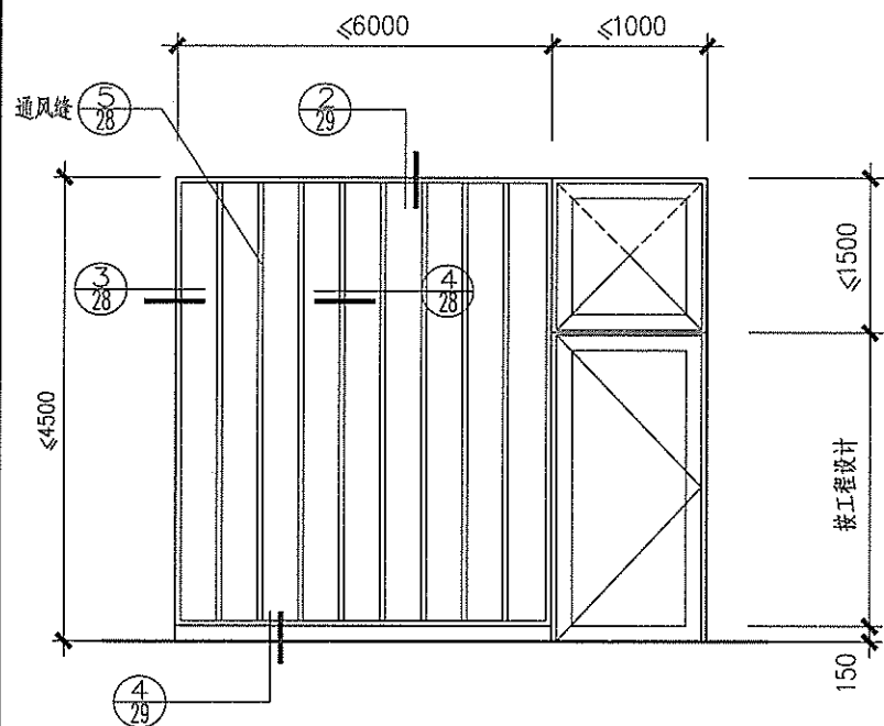
① 单层全玻带门隔断立面图
