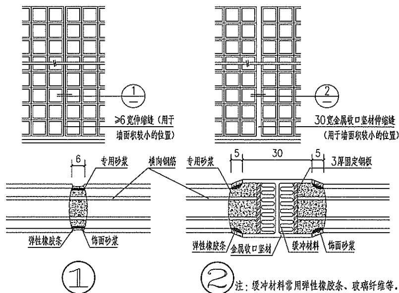
玻璃砖隔断变形缝做法
