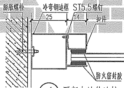
④ 隔断与墙体连接
