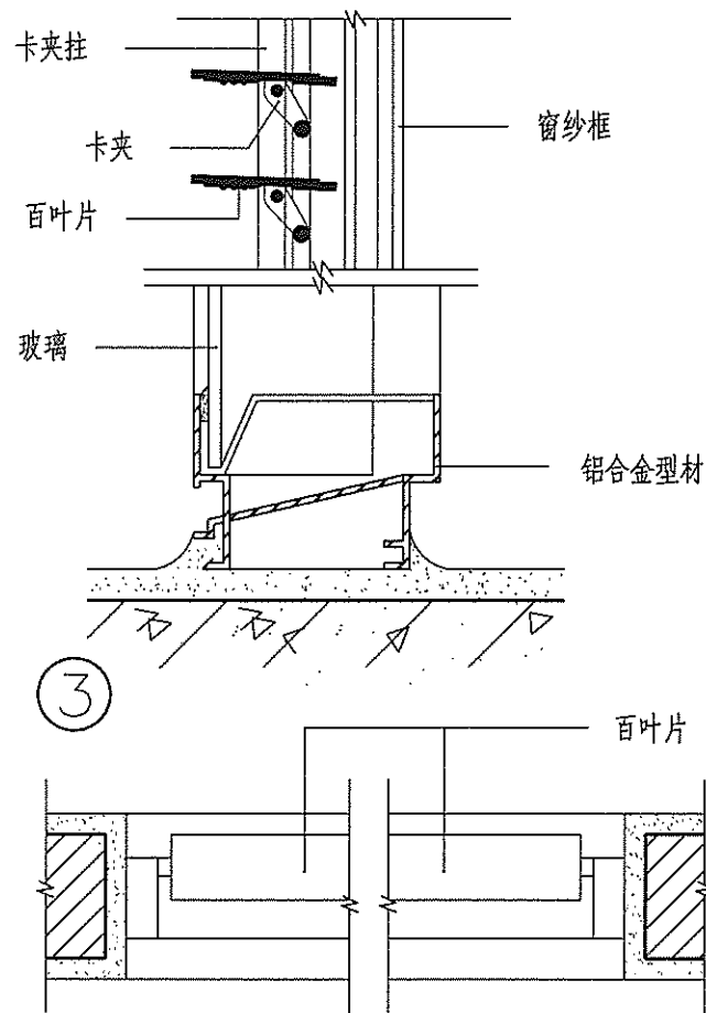
Ⓐ 玻璃活动百叶隔断平面示意图
