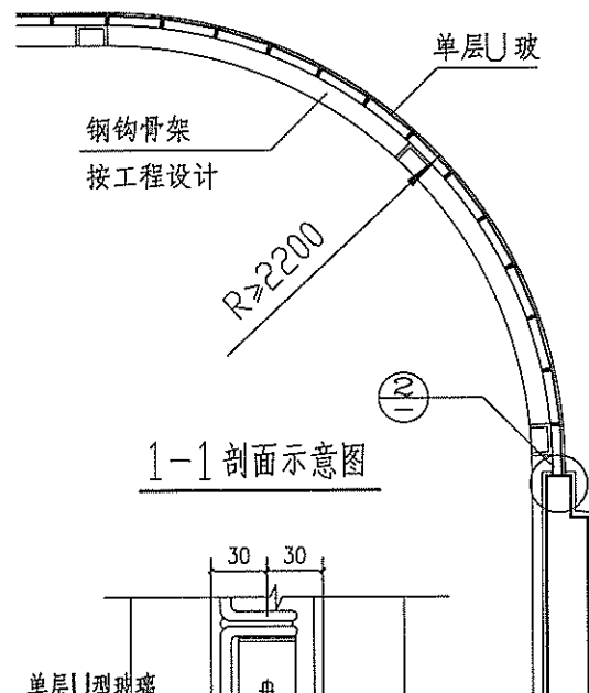
铝或不锈钢压条
