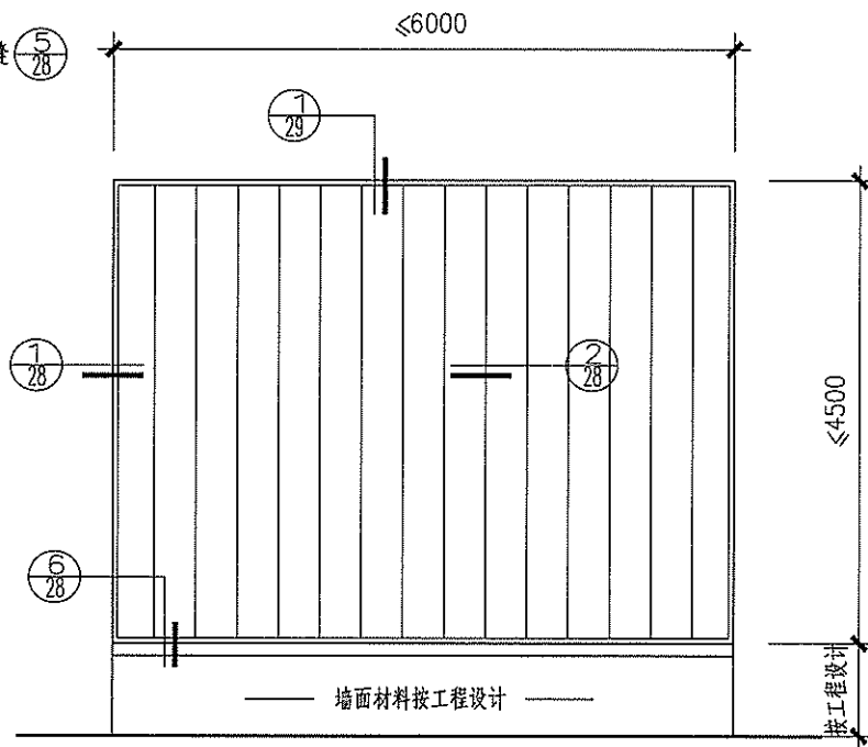
③ 双层半玻隔断立面图
