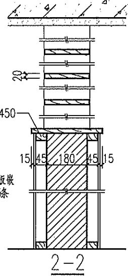
博古架木隔断 (一)
