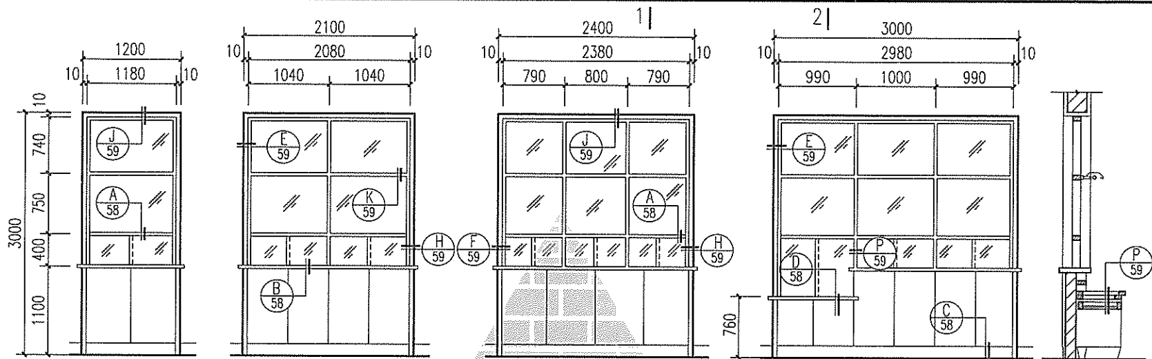
④ 外立面 (含无障碍窗口) 1-1
