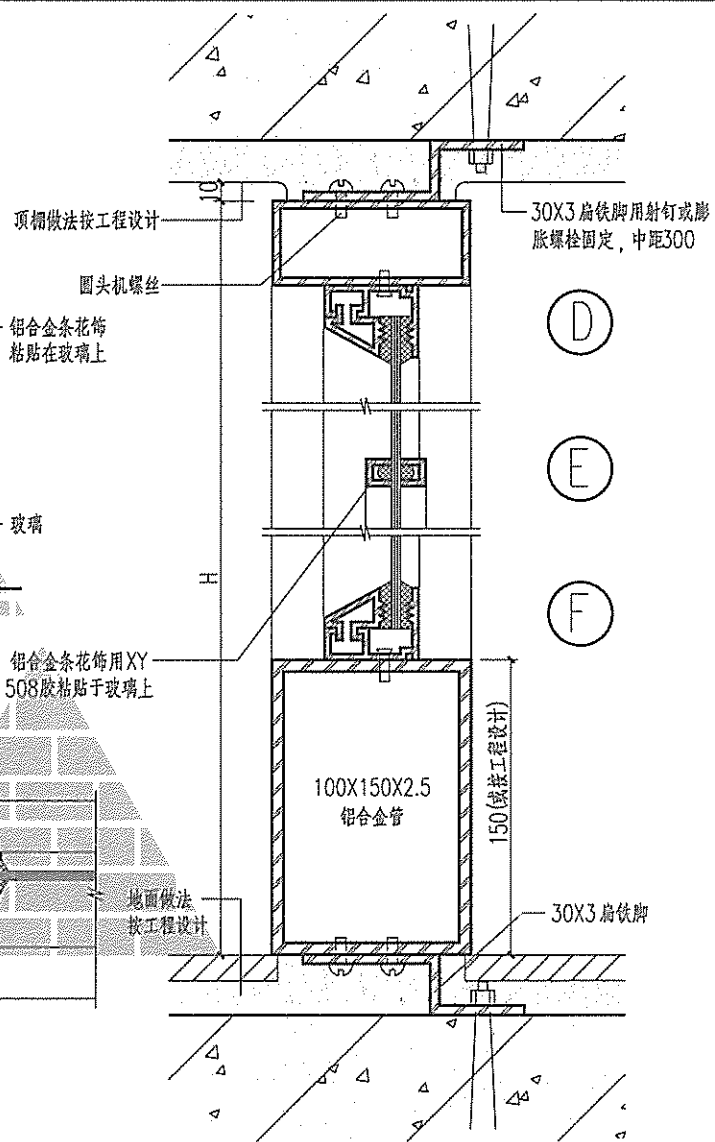
铝合金隔断(五)
