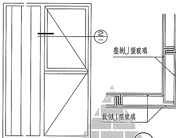
全玻隔墙—门立面图
