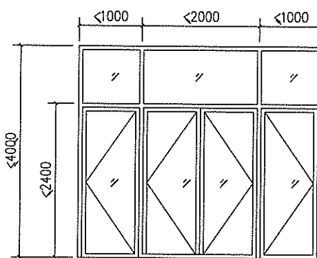
基本单元2与平开门组合立面示意图2
