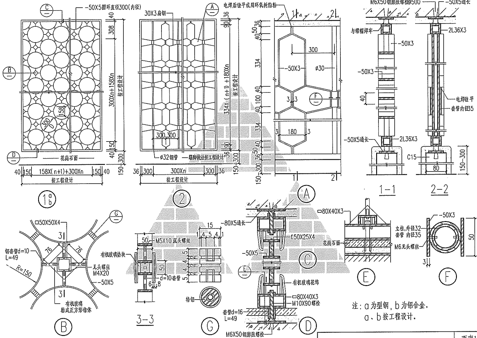
钢、铝合金花饰隔断
