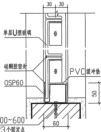
U型玻璃隔断 (九)
