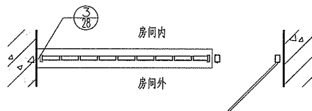
② 单层全玻带门隔断平面图
