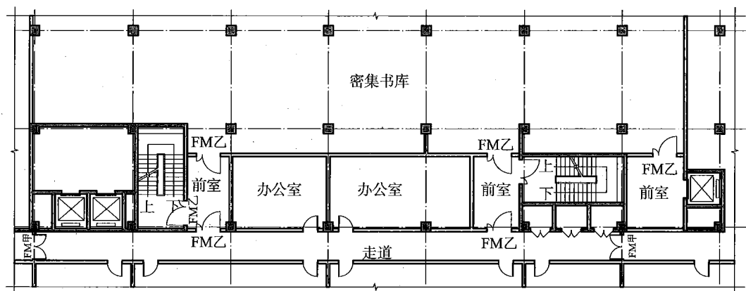
图2 地下书库和设备层
