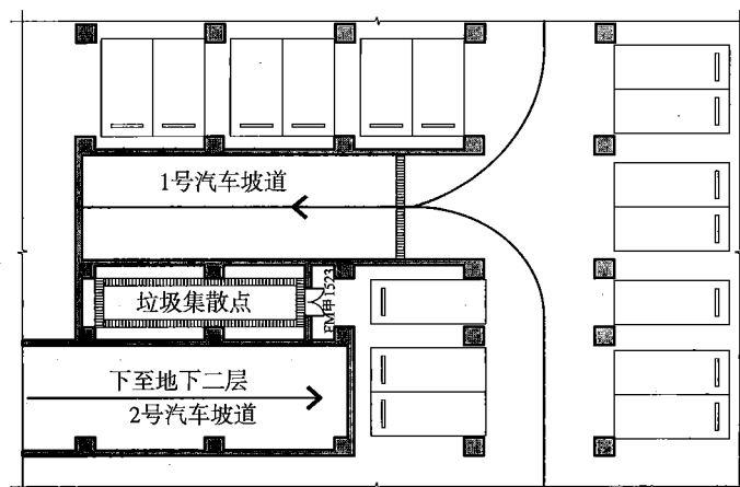
图 2 地下汽车库防火分区内垃圾集散点
