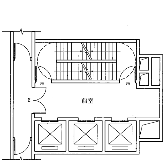
图 3 高层住宅 2 户（前室间门可取消）
