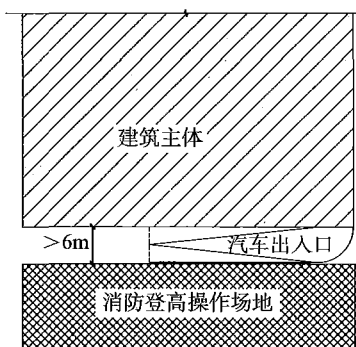
图2 坡道与消防车登高操作场地平行
