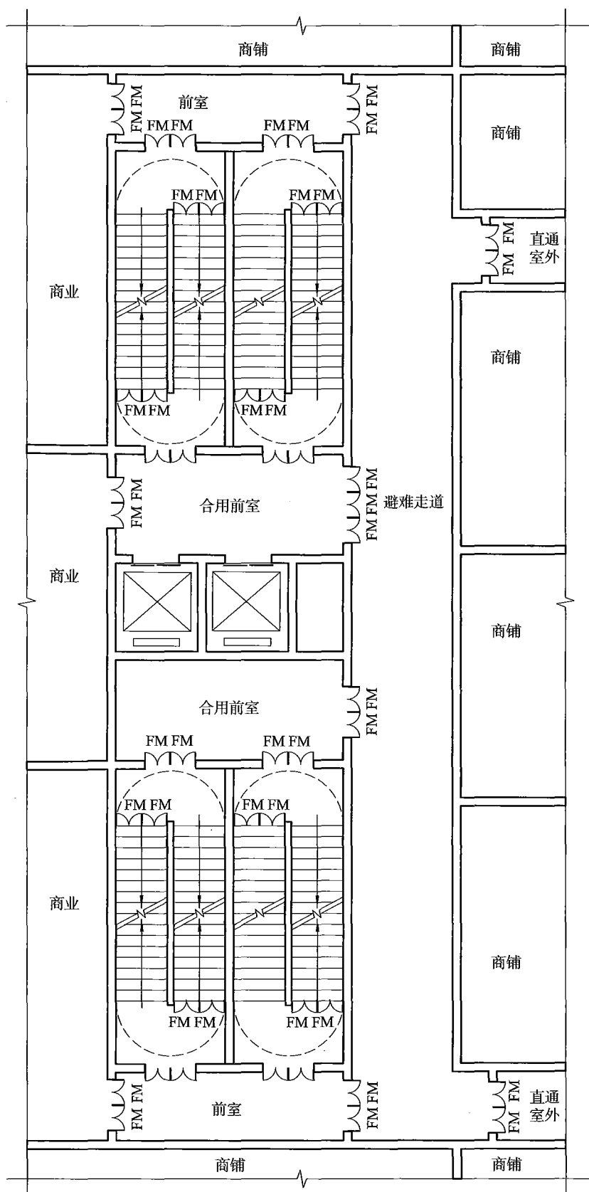
图2 高层综合楼首层平面局部图
