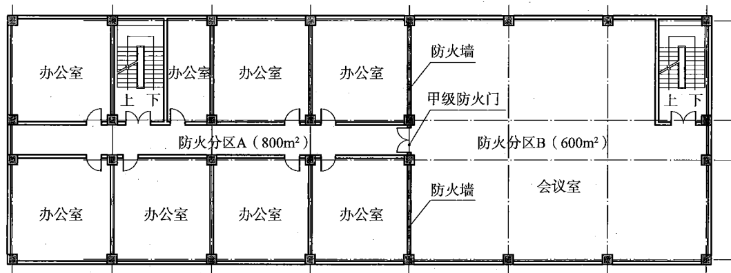
图1 某办公建筑8层平面图
