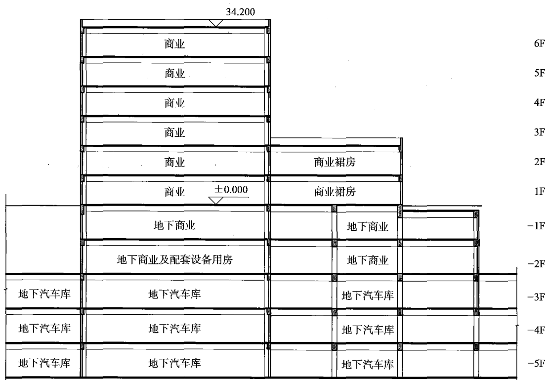
图1 含地下汽车库的综合建筑剖面示意图
