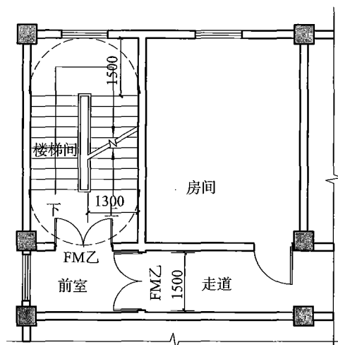
图 1 防烟楼梯间平面局部图
