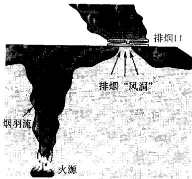
图 15 排烟口的最高临界排烟量示意图
