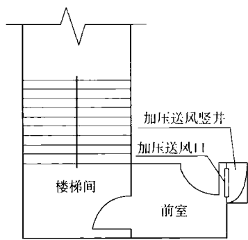
图 1 挡住加压送风口的疏散门
