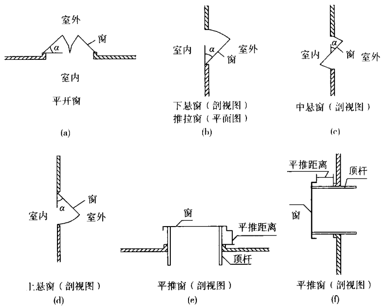
图 6 可开启外窗的示意图
