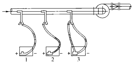
图 20 吸入段毕托管与倾斜式微压计的连接方法 1—全负压;2—静负压;3—动压
