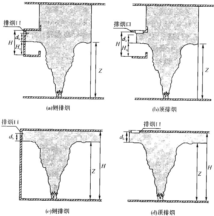
图 16 排烟口设置位置参考图
