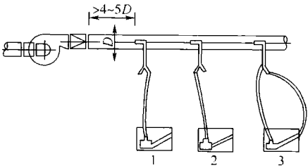
图 21 压出段毕托管与倾斜式微压计的连接方法 1—全正压；2—静正压；3—动压
