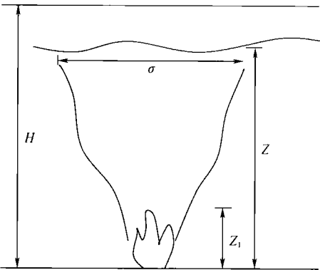
图 10 轴对称型烟羽流
