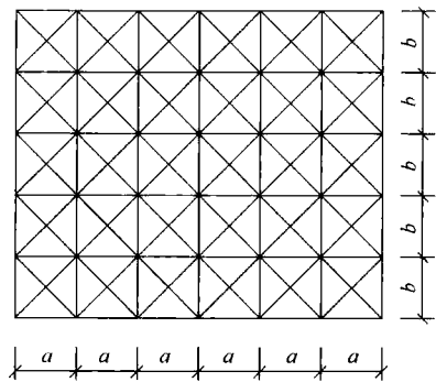
图 17 矩形风管测点布置图
