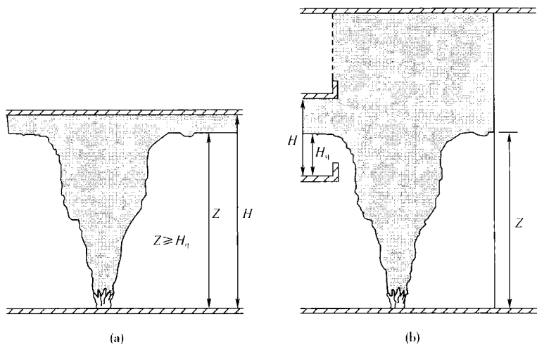
图 9 最小清晰高度示意图
