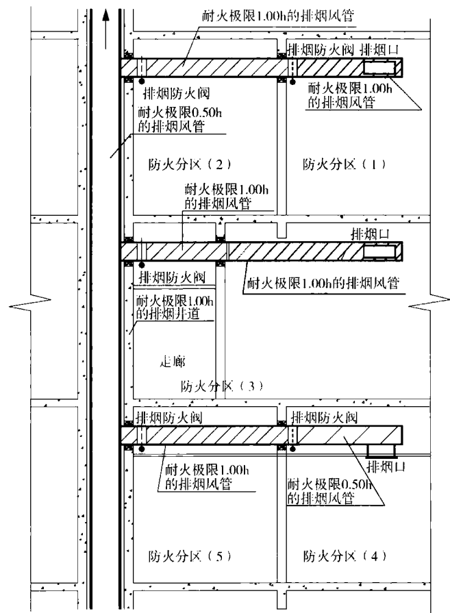
图 7 排烟管道布置示意图
