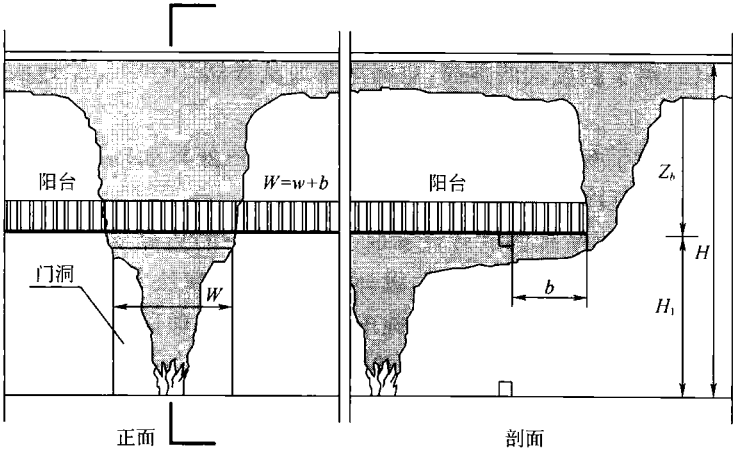
图 11 阳台溢出型烟羽流
