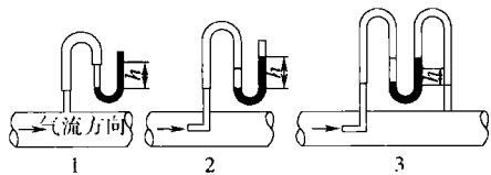
图 19 用 U 形管压力计测定风压 1—静压;2—全压;3—动压
