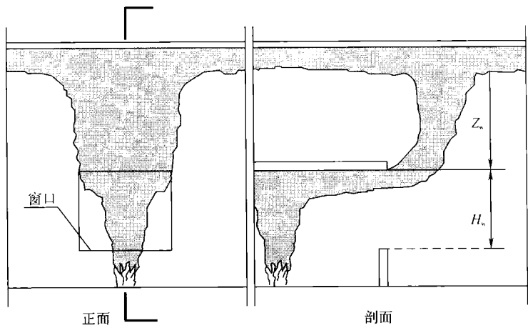
图 12 窗口溢出型烟羽流
