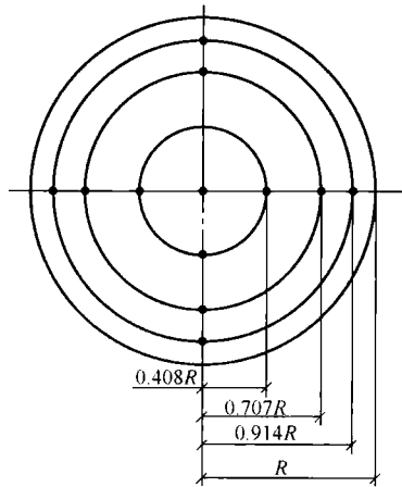
图 18 圆形风管测点布置图
