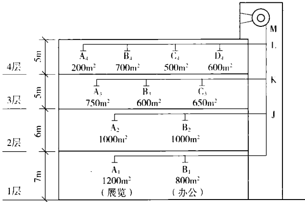
图 8 排烟系统示意图
